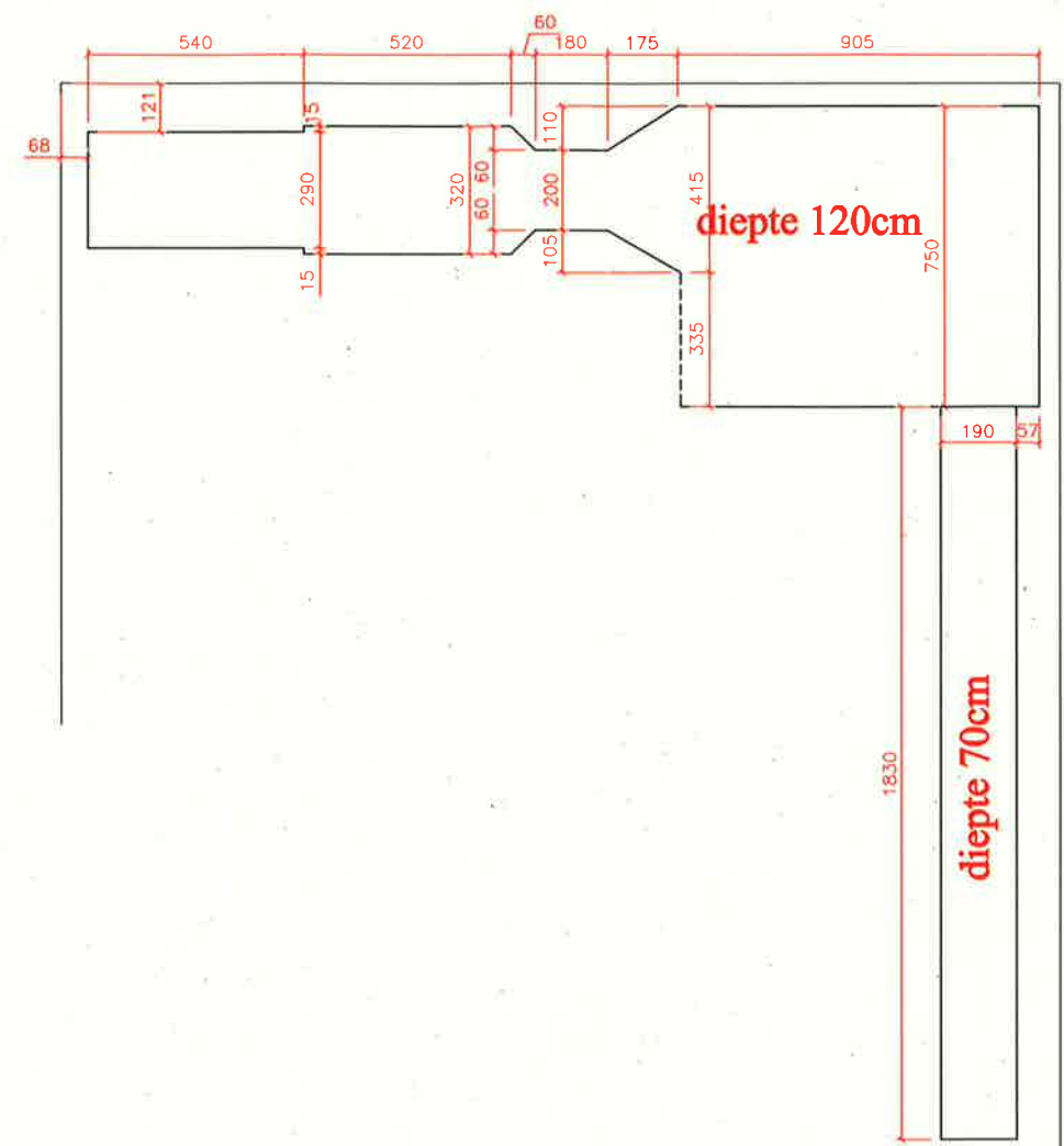
AFMETINGEN BETONKUIP LANDINGSKUIP / TRAMPOLINEBAAN
